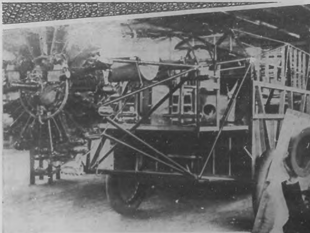
En los talleres de la casa Fokker, en Amsterdam, Holanda, se está construyendo el monoplane que el comandante Byrd utilizará en su viaje al Polo antártico. La foto muestra el motor y algunas de las partes principales del aparato.
